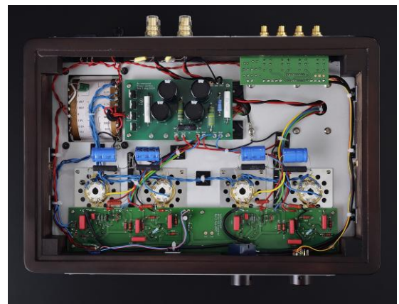
内部配線の様子 手配線とプリント基板を適材適所に配備 通常の2倍の銅箔厚を使用
